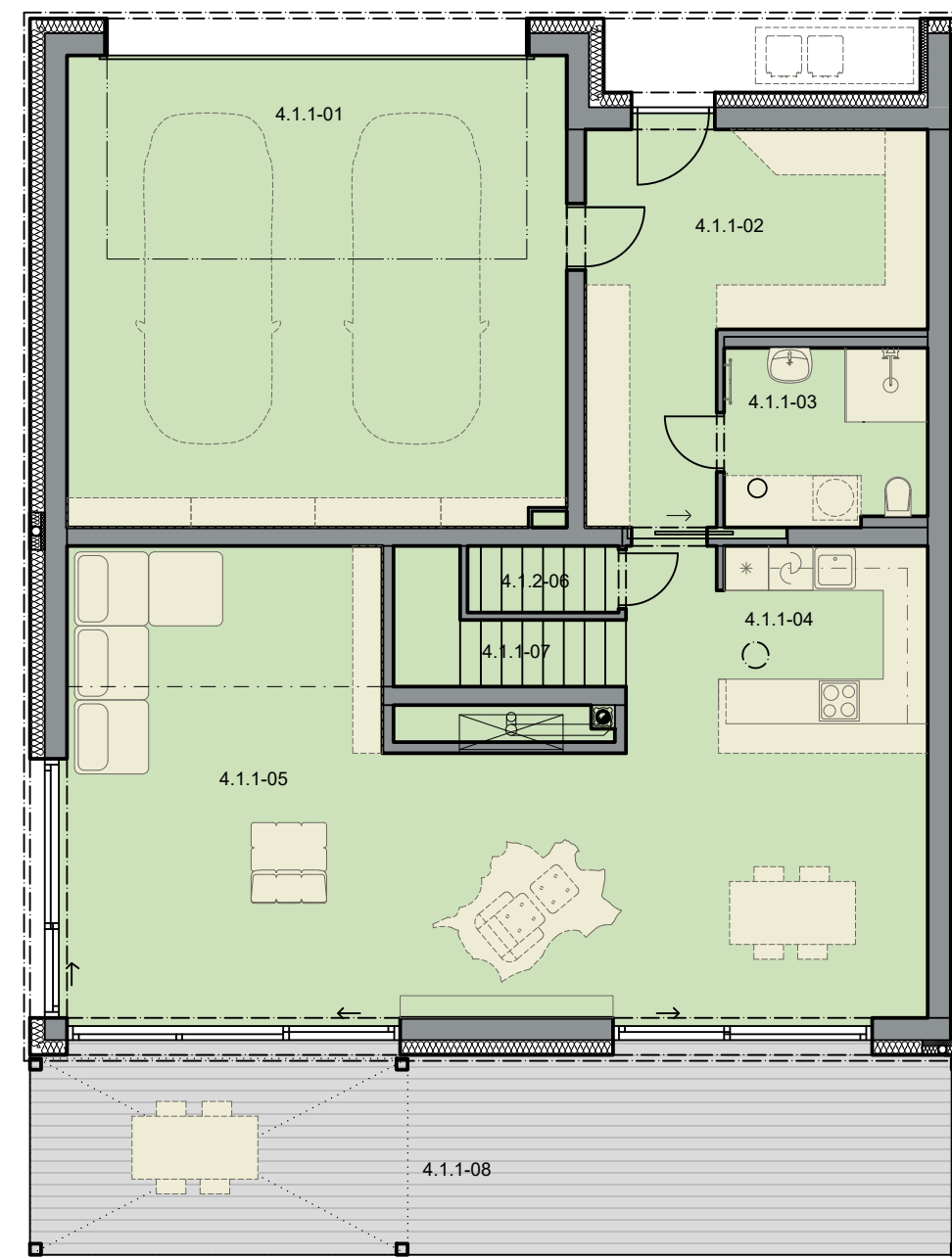
PŮDORYS 1NP 1:100
