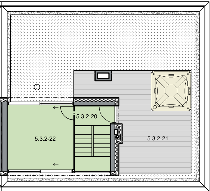
PŮDORYS 3NP 1:150
