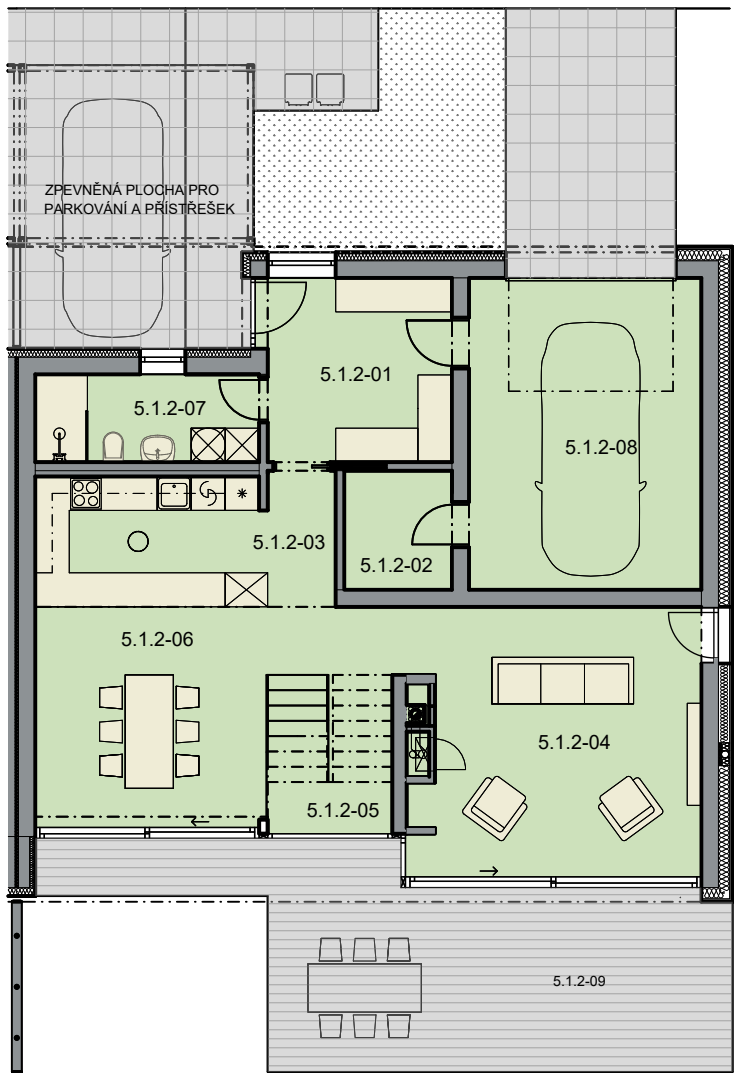
PŮDORYS 1NP 1:150
