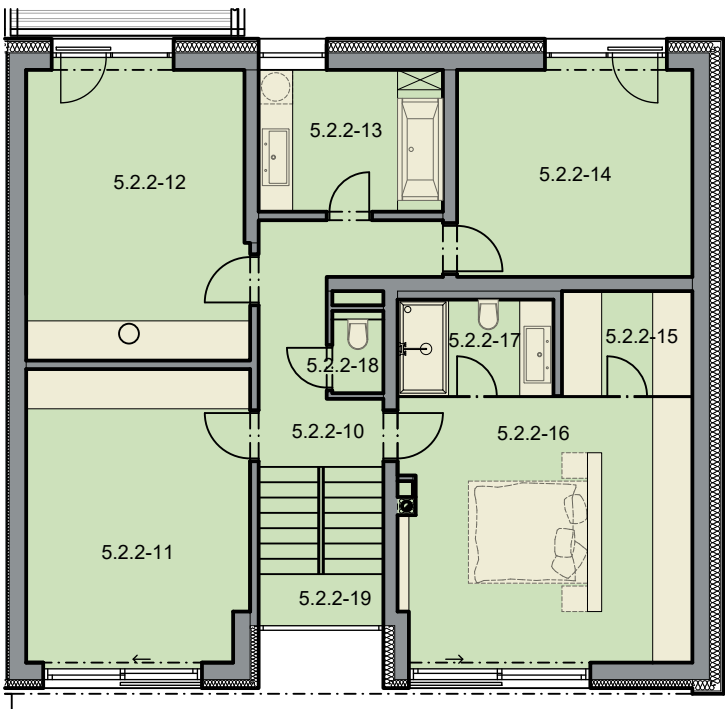
PŮDORYS 2NP 1:150
