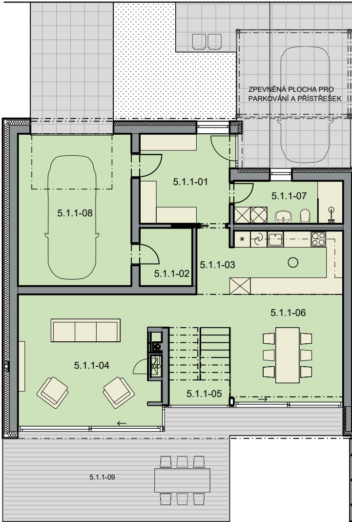
PŮDORYS 1NP 1:150
